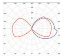
Modèle 1 avec cache lampe E27 (2450 lm) Flux sortant - 1180 lm
