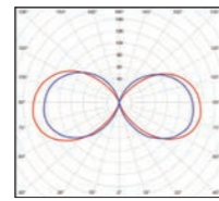
Modèles 1 à 4 sans cache lampe E27 (2450 lm) Flux sortant - 2350 lm
